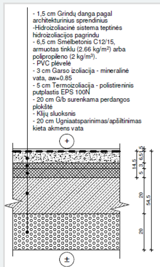
Sanitarinio mazgo grindų įrengimo schema pirmojo aukšto (butai)
